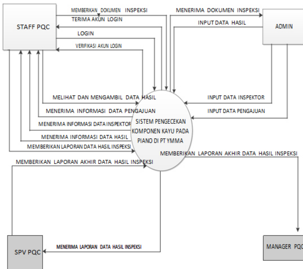
Gambar 1: Diagram Konteks
